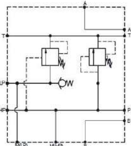
ESQUEMA HIDRÁULICO
