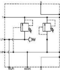
ESQUEMA HIDRÁULICO
