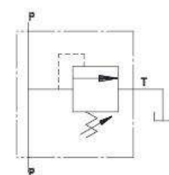
ESQUEMA HIDRÁULICO
