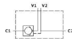
ESQUEMA HIDRÁULICO
