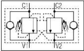
ESQUEMA HIDRÁULICO
