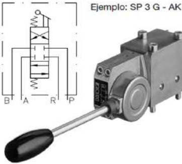
Versión para montaje sobre placa
