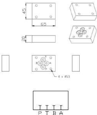
CETOP 3 - NG6
