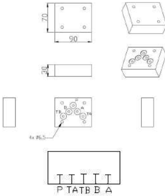
CETOP 5 - NG10
