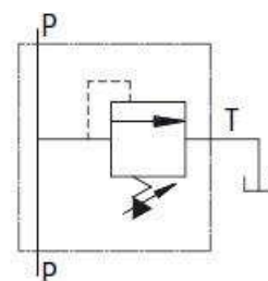
ESQUEMA HIDRÁULICO
